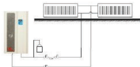
Caldaia EKW-AsBN come fonte di calore autonoma
