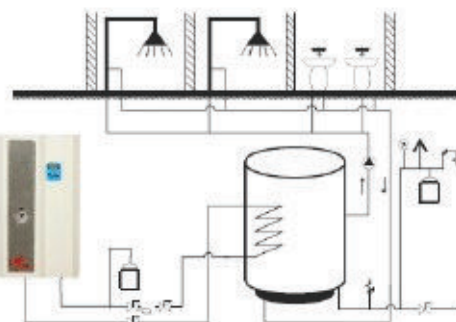
Caldaia EKW-AsBN con il serbatoio dell'acqua calda riscaldamento di grosse quantità d'acqua in poco tempo
