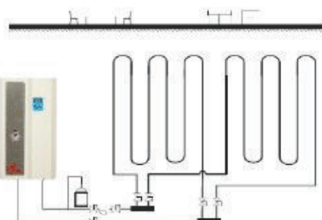
(Temperatura di lavoro della caldaia massima 40°C) Caldaia EKW-AsBN nell'impianto di riscaldamento da pavimento
